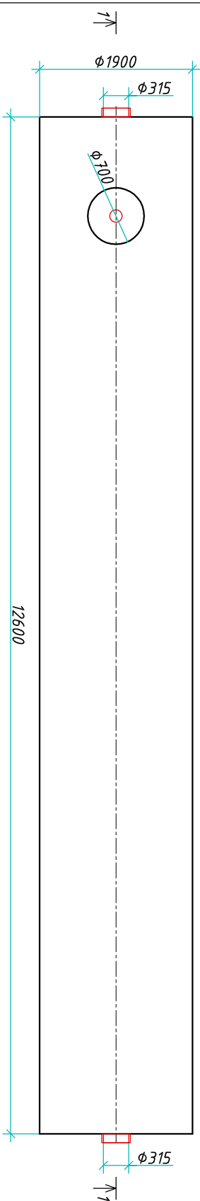
Вид сверху
