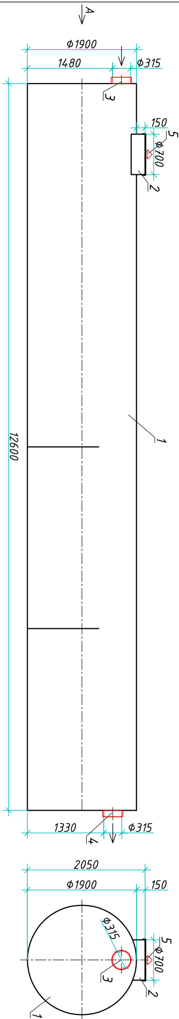
Разрез 1-1
